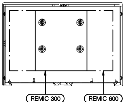
Fixation des jeux de barres REMIC 300 et REMIC 600 ( 1 configuration )
