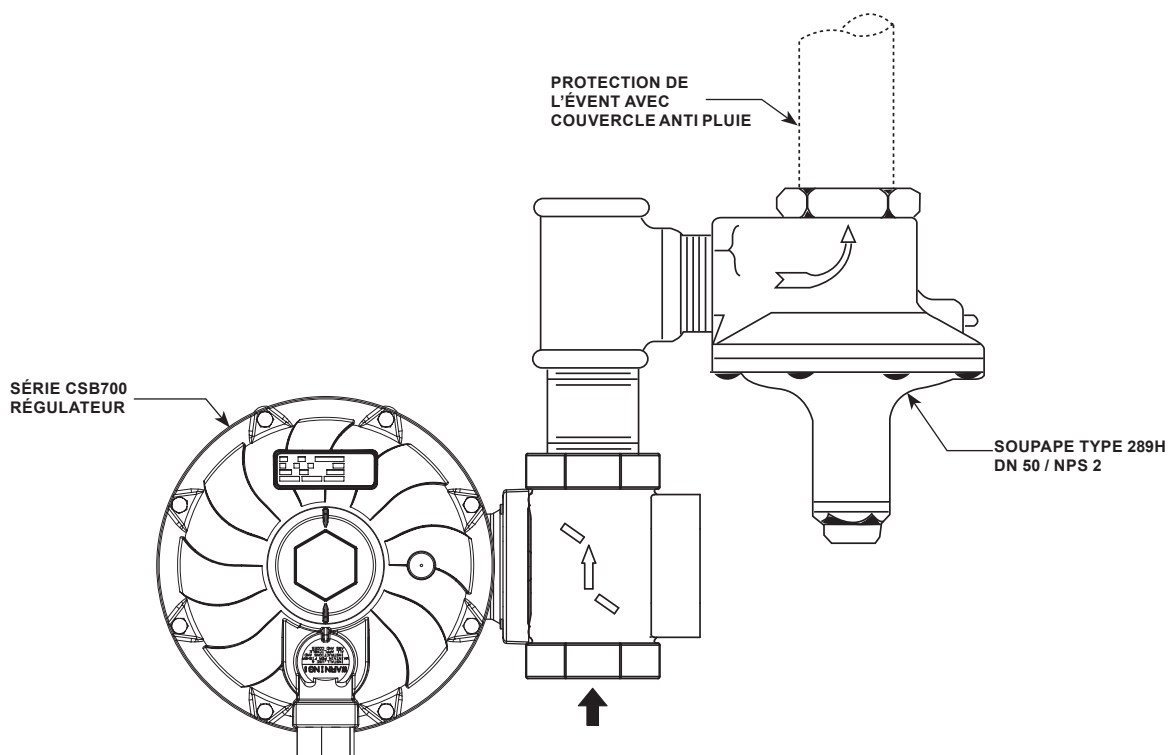
Figure 5. Série CSB700 Régulateur avec Installation Évnt Vers le Bas et Type 289H Soupape à Grande Capacité
