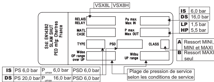
PLAQUE SIGNALÉTIQUE DU RELAIS DÉCLENCEUR
