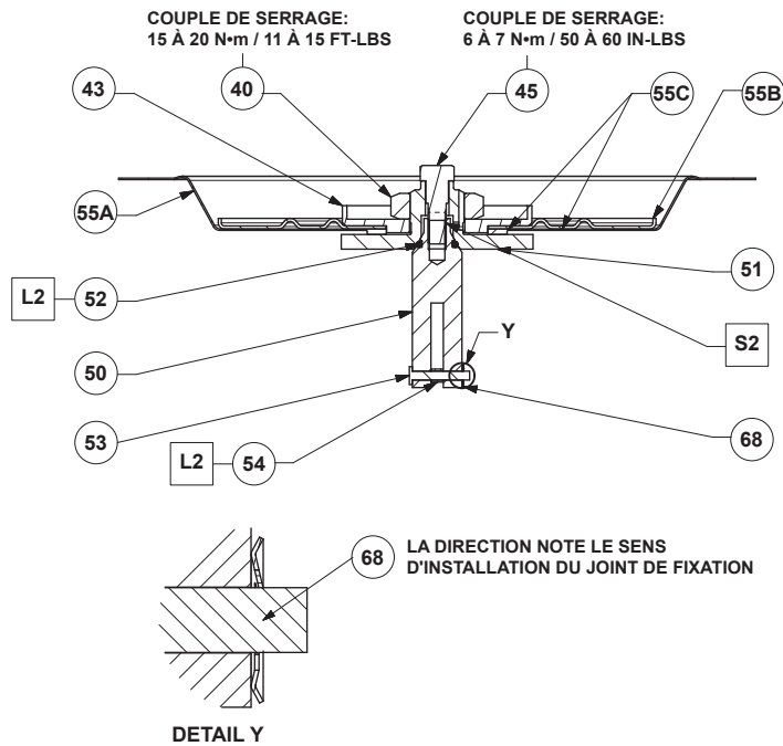
ENSEMBLE MEMBRANE POUR LES TYPES CSB700 ET CSB720 (61 À 570 mbar / 0.9 À 8.3 psig) SANS SOUPAPE
