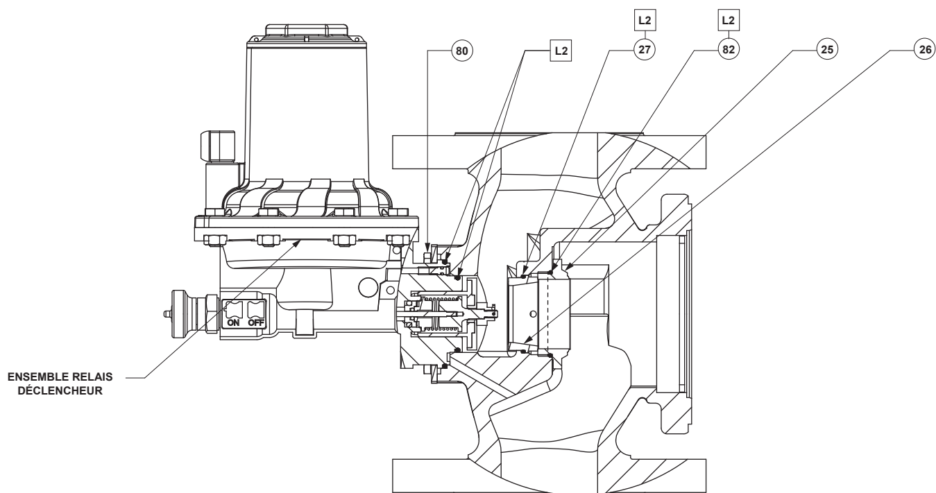
ORIFICE ET ENSEMBLE RELAIS DÉCLENCHEUR
