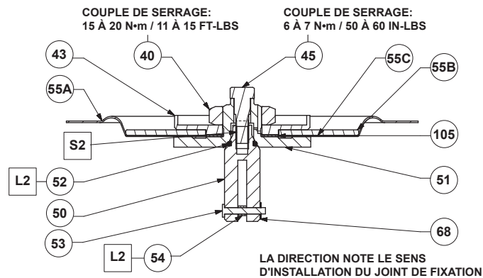
ENSEMBLE MEMBRANE POUR LE TYPE CSB750 SANS SOUPAPE
